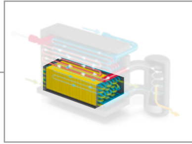
Échangeur de chaleur air/frigorigène avec accumulateur frigorigère (en jaune)
