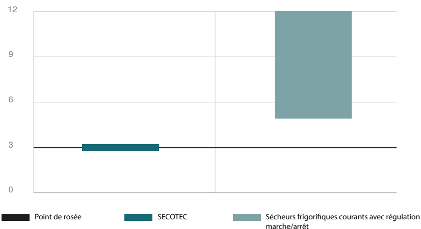
Degré de séchage exprimé en point de rosée moyen en °C
